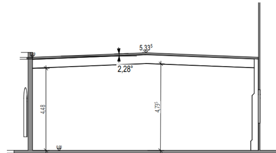
Ansicht Nord-Westen
